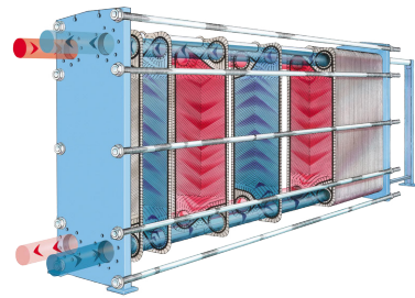
可拆板式冷却器
