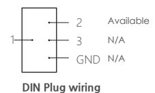
DIN Plug wiring
