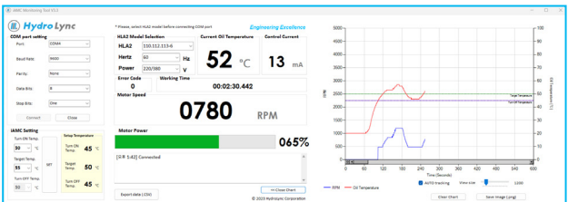
iAMC软件
