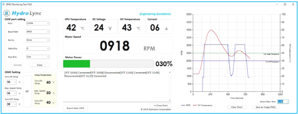
监测软件
