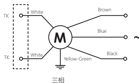
电机布线
