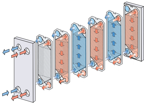
热流体和冷流体的流动方向
