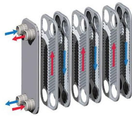
钎焊板式冷却器
