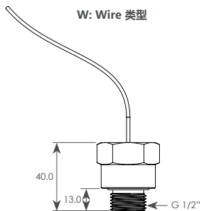
W: Wire 类型
